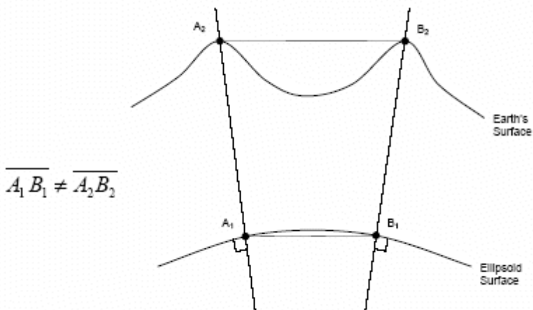
Рисунок 1. Расхождение нормалей к поверхности эллипсоида
